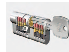
Key One X-pert Wkładka pojedyncza w profilu podstawowym
