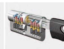
Key Tec RPE Innowacyjny system bazowy dla wkładek pojedynczych i w identycznym kodowaniu
